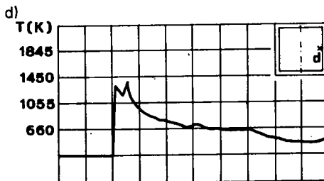
Rys.3. Rozkład temperatury w płomieniu gazowo-pyłowo-powietrznym, w różnych odległościach od ścianki kanału (pył węgla brunatnego). a) w osi kanału, b) 25 mm od ścianki, c) 6 mm od ścianki, d) 2 mm od ścianki
